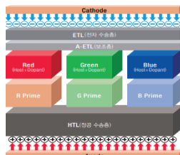
OLED 패널 구조
